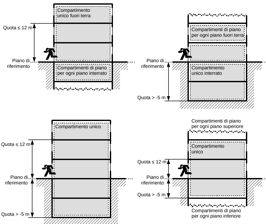
Illustrazione S.3-1: Esempi di compartmentazione multipiano, in sezione
